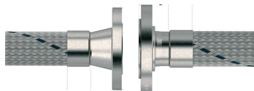
ASME B16.5 Flange (Swivel/Fixed)
